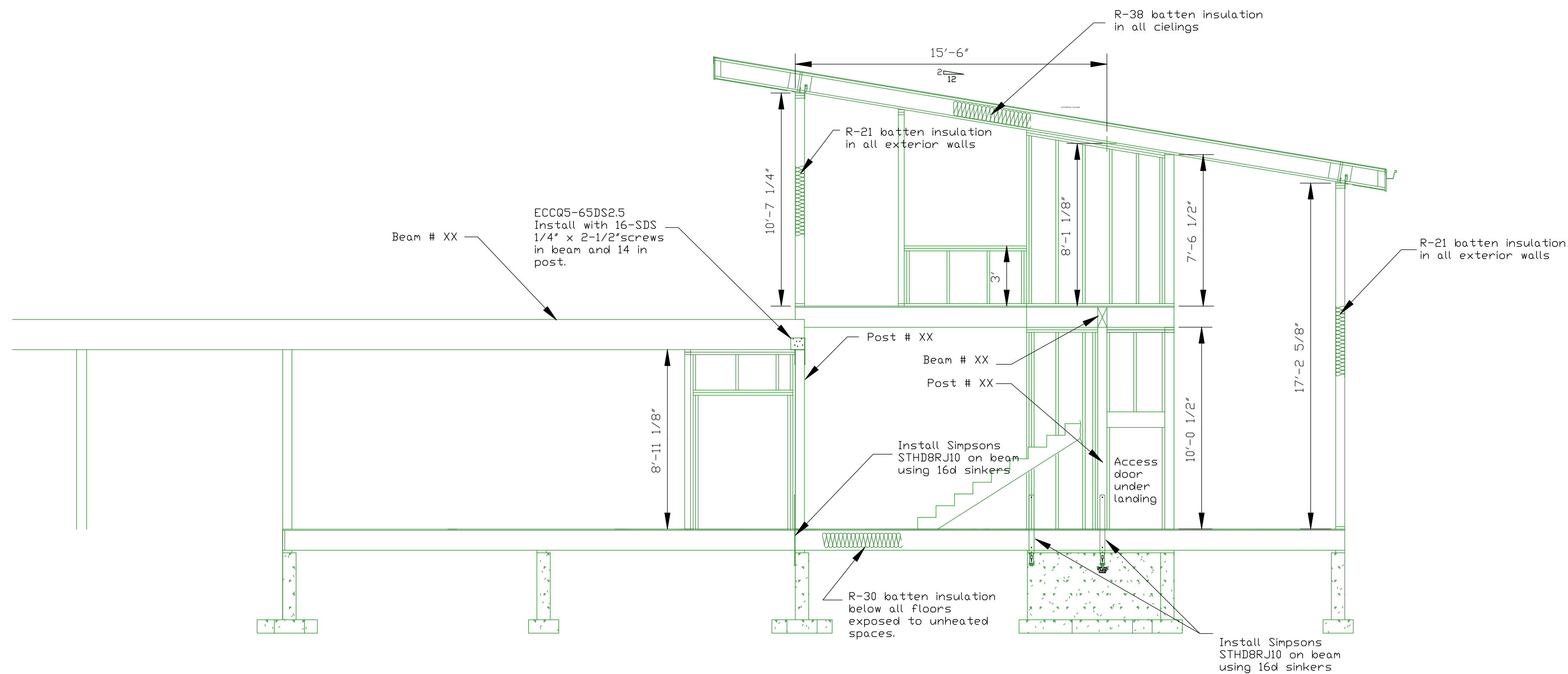
Section XX Scale: 1/4" = 1'- 0"
