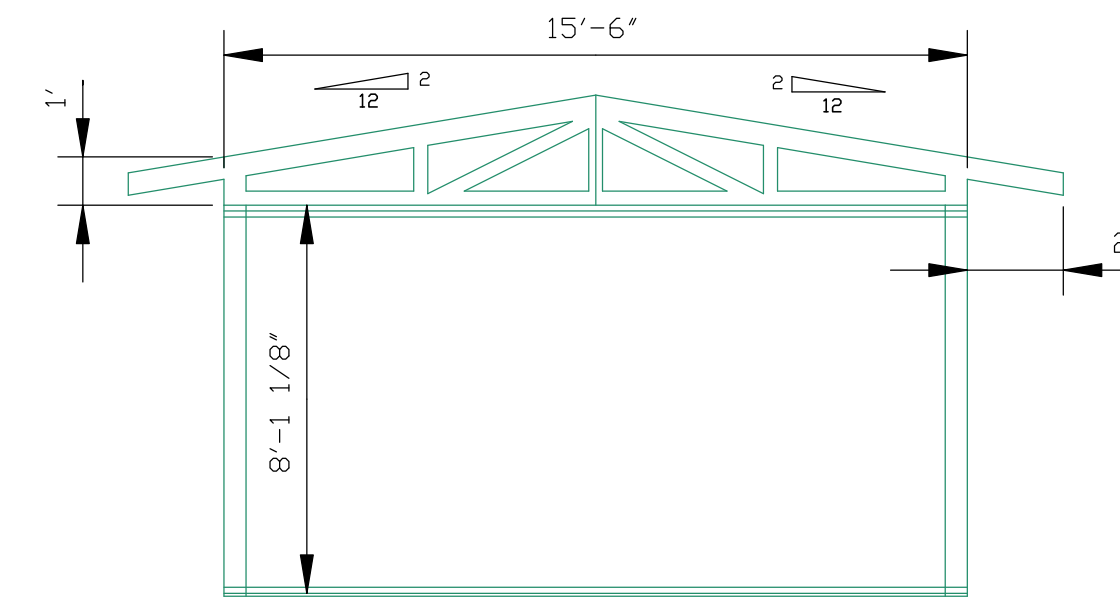
Section XX Scale: 1/4" = 1'- 0"
