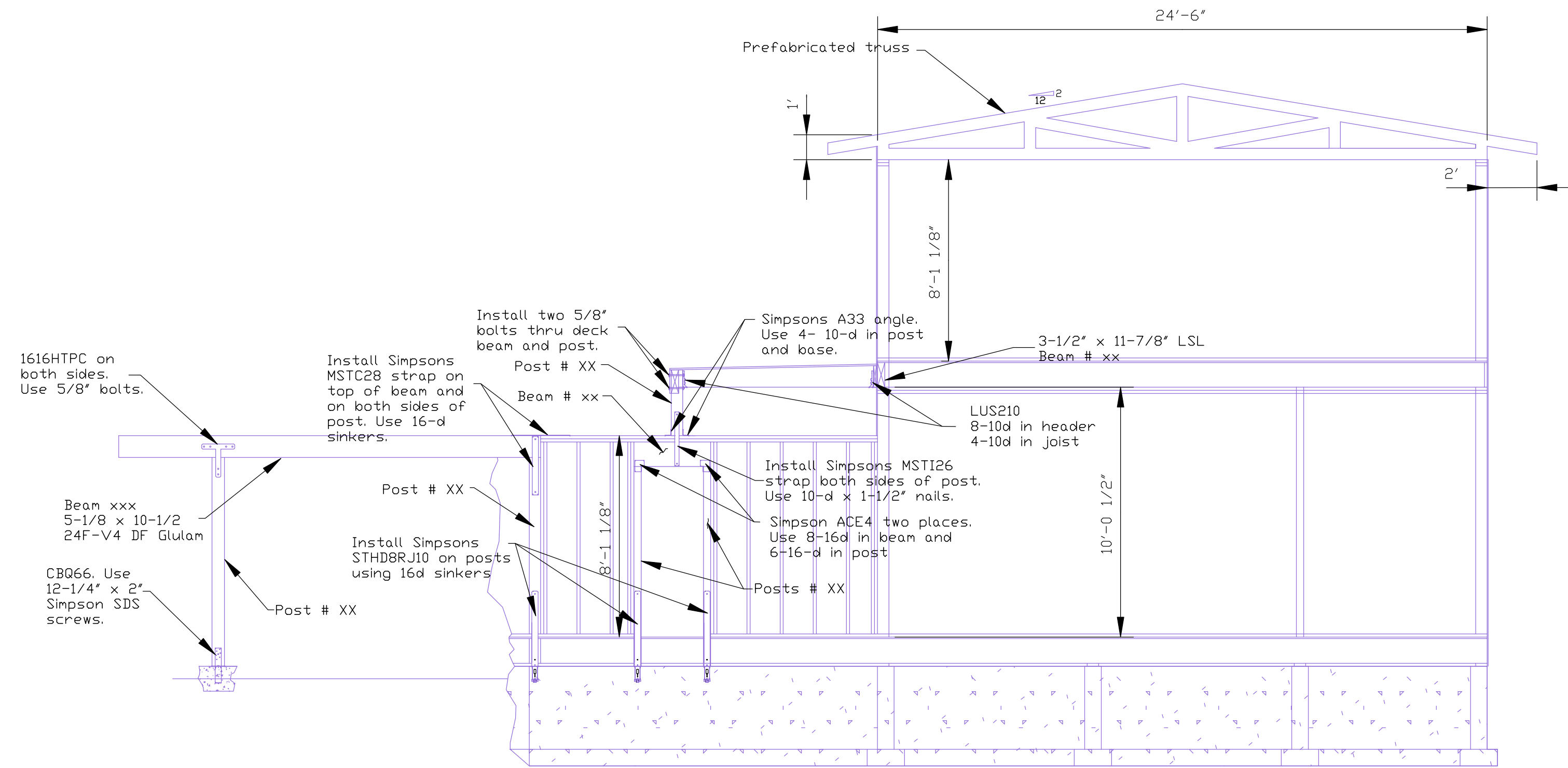
Section XX Scale: 1/4" = 1'- 0"
