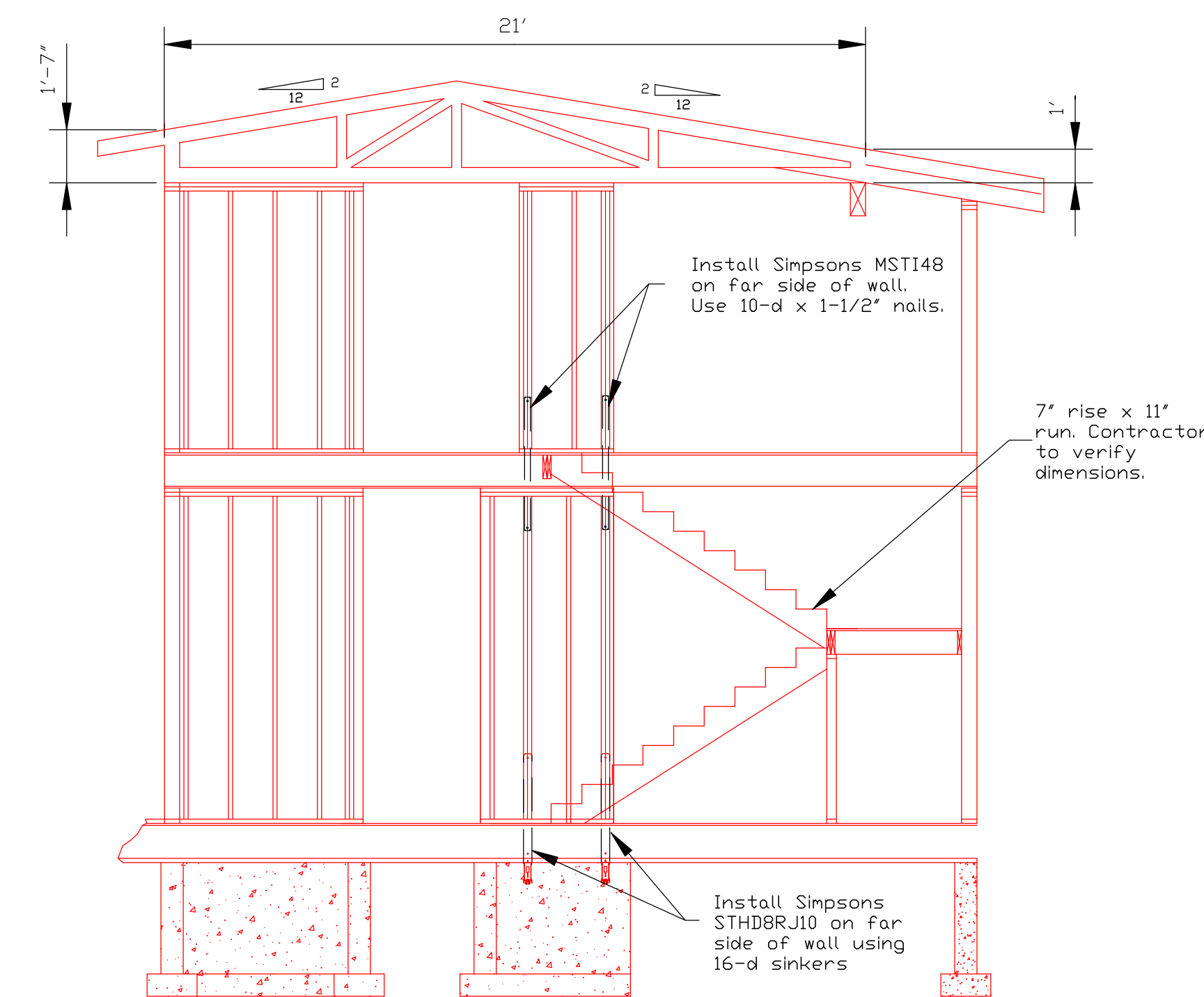
Section XX Scale: 1/4" = 1'- 0"
